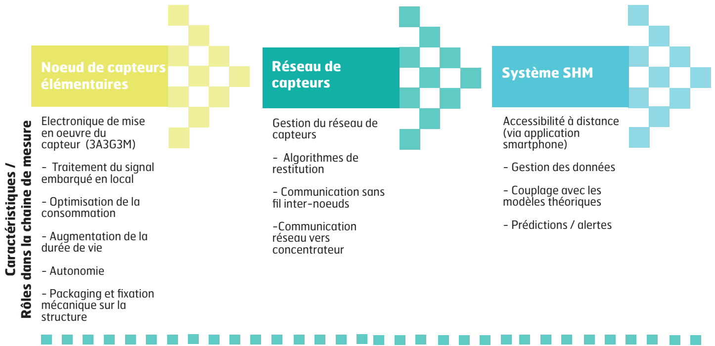
FIGURE 3 : Description de la chaîne de mesure du SHM 2
